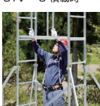
上階用布枠により、先 行して手すりが取付け られ、安全帯をかけな がら、安全に組立てが 可能に。
